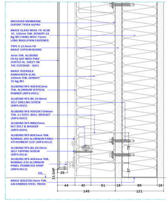
DT-8 2246 SCALE 1:2
