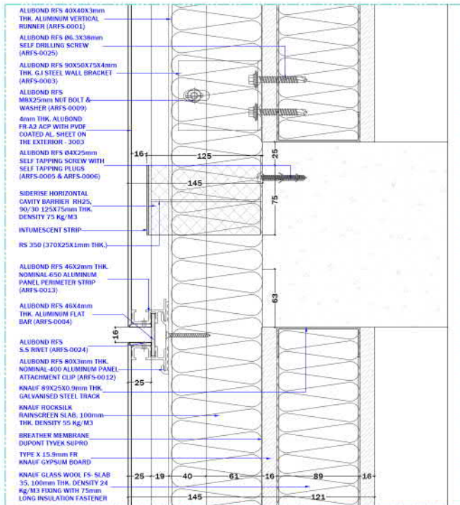
DT-9 2246 SCALE 1:2
